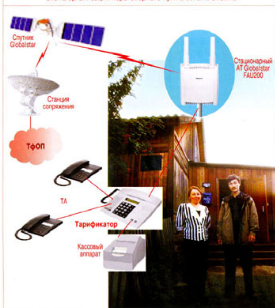
Схема организации переговорного пункта связи в Сизиме
